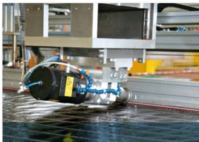
Saldatura ultrasuoni piastra captante
